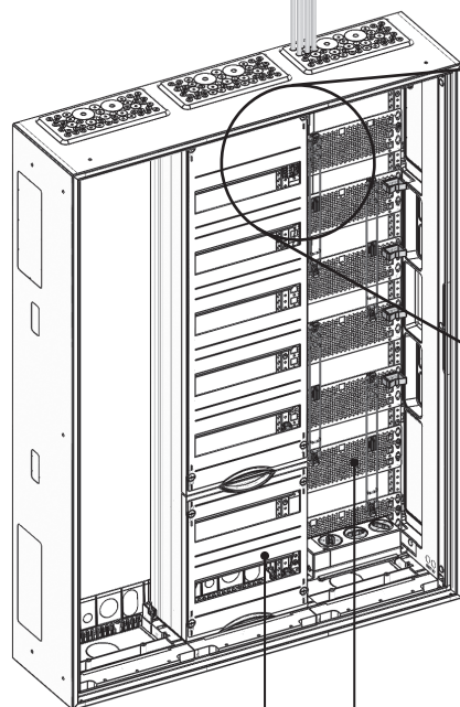
Verteilerfeld Distribution Panel
