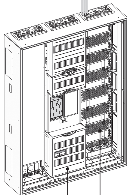
Zählerfeld Meter Panel
