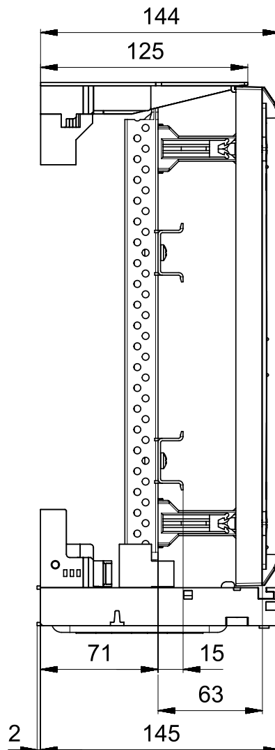
Maße CombiLine-MP für Aufbau von CombiLine-Module auf der vorderen Ebene
