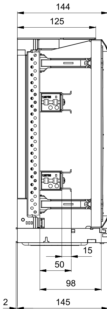
Maße CombiLine-MP für Aufbau Zählerplatte und Mediafelder auf der hinteren Ebene
