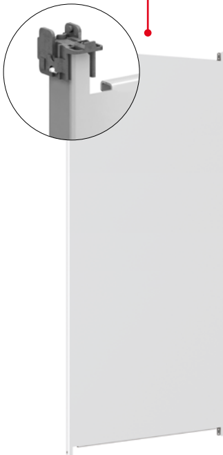
Einbau Montageplatte* Ausbau für die Steuerungstechnik mit Montageplatte
