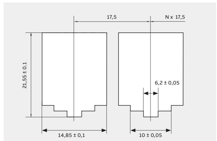
Maße Aussparungen E-DAT-Module
