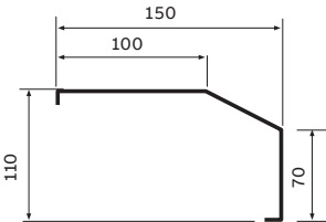
Schnittdarstellung Rangierblende
