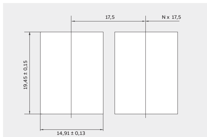
Maße Aussparungen Keystone-Module
