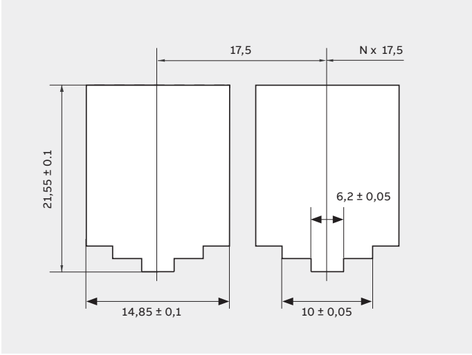
Maße Aussparungen E-DAT-Module
